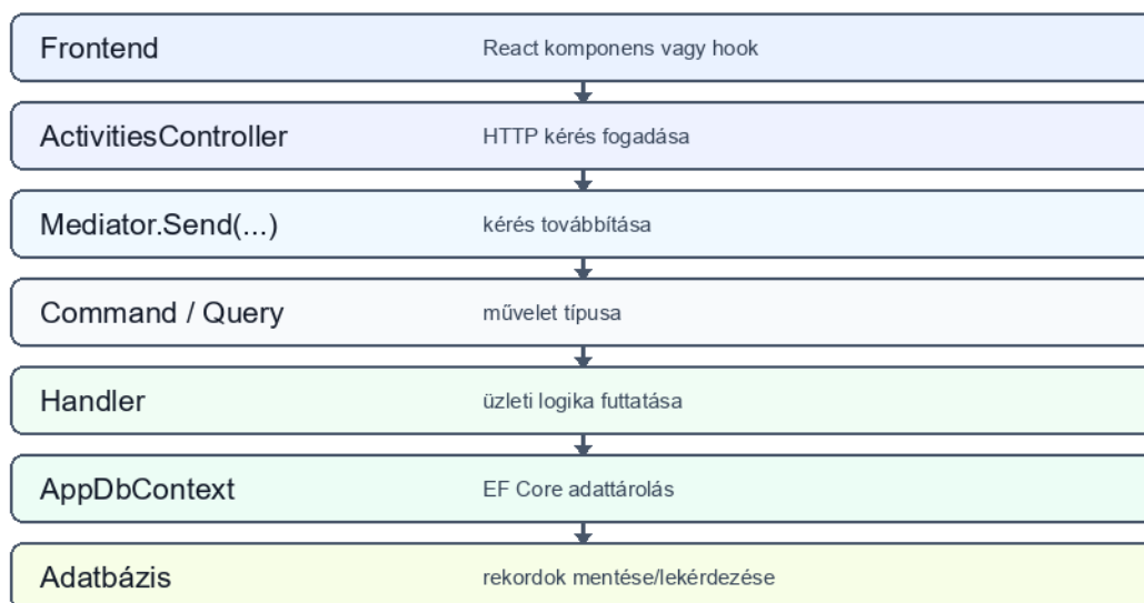
16. ábra: A MediatR közvetítő szerepe a frontend és az adatbázis között
